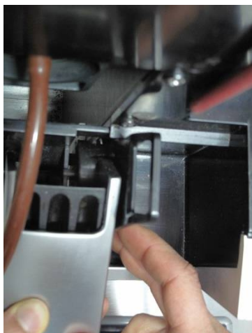
Wsuń wylewkę pod obie prowadnice i załóż na miejsce
